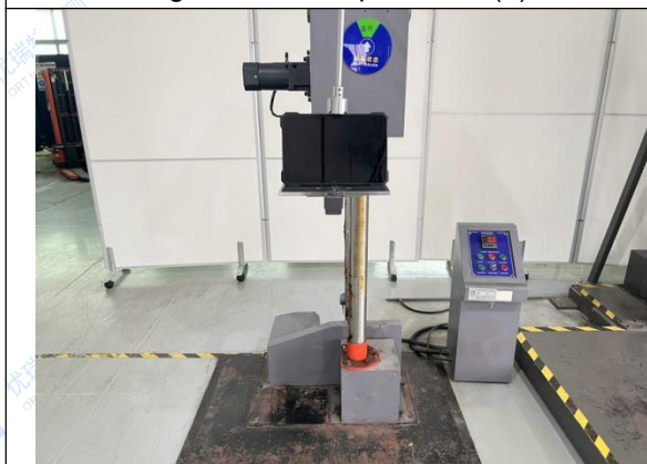
Fig.68 Test setup- Edge (1)
