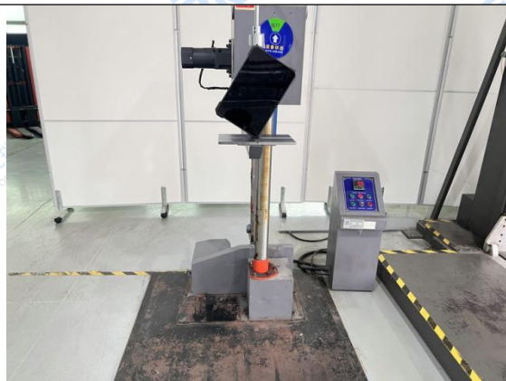
Fig.78 Test setup- Edge (11)
