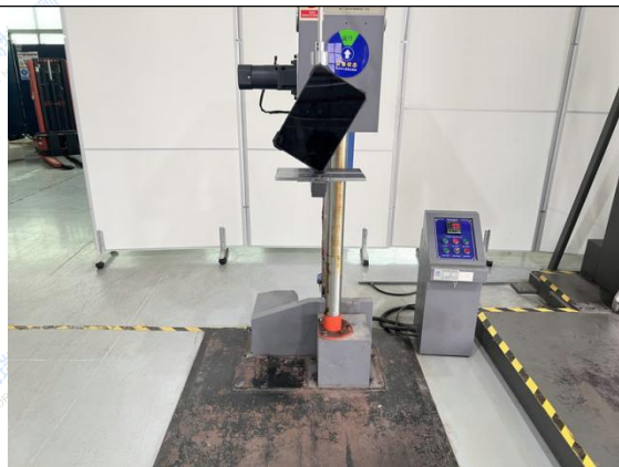
Fig.76 Test setup- Edge (9)
