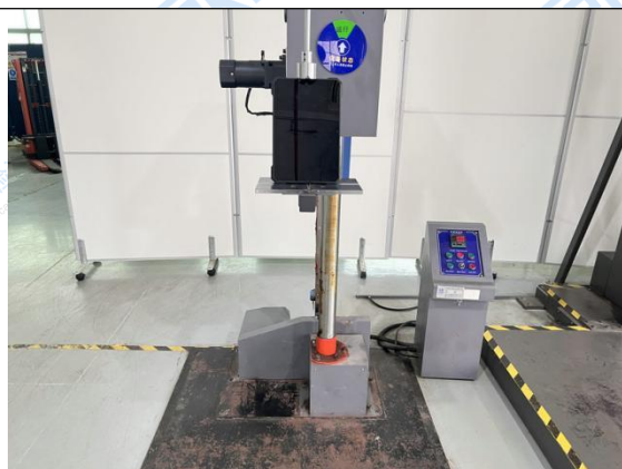
Fig.73 Test setup- Edge (6)
