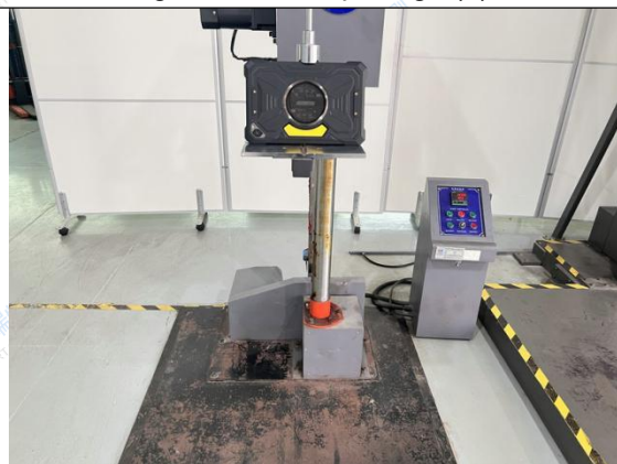
Fig.71 Test setup- Edge (4)
